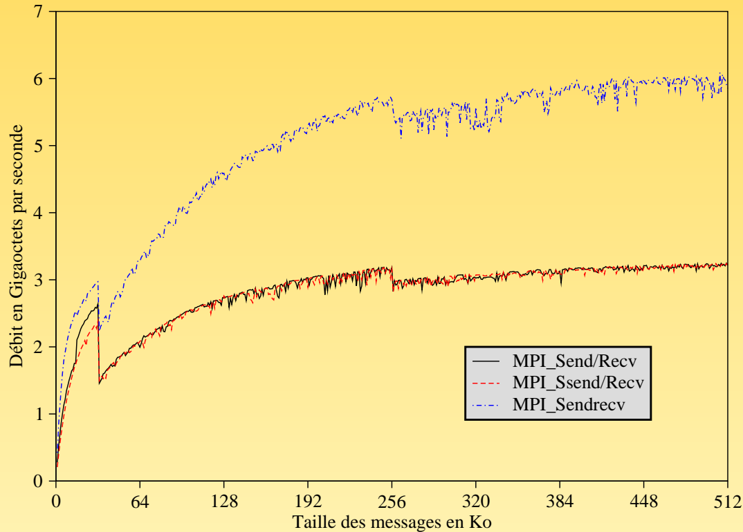
Débits des communications point à point intra-noeud sur la machine IBM P6 (valeur par défaut de MP_EAGER_LIMIT)
