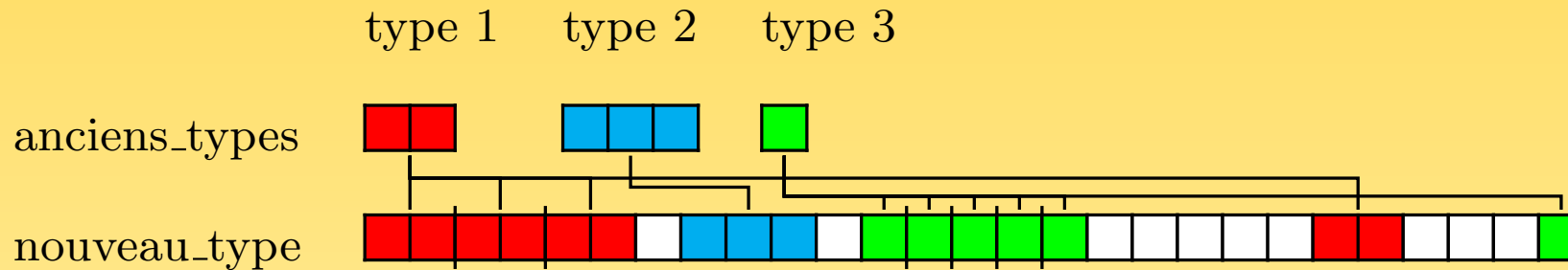
FIG. 31 – Le constructeur MPI_TYPE_CREATE_STRUCT
