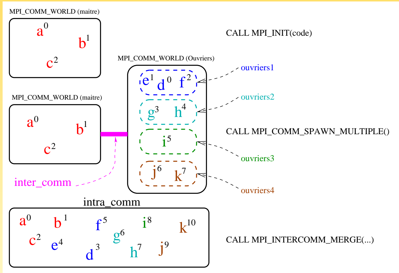
FIG. 84 – Utilisation de MPI_COMM_SPAWN_MULTIPLE()
