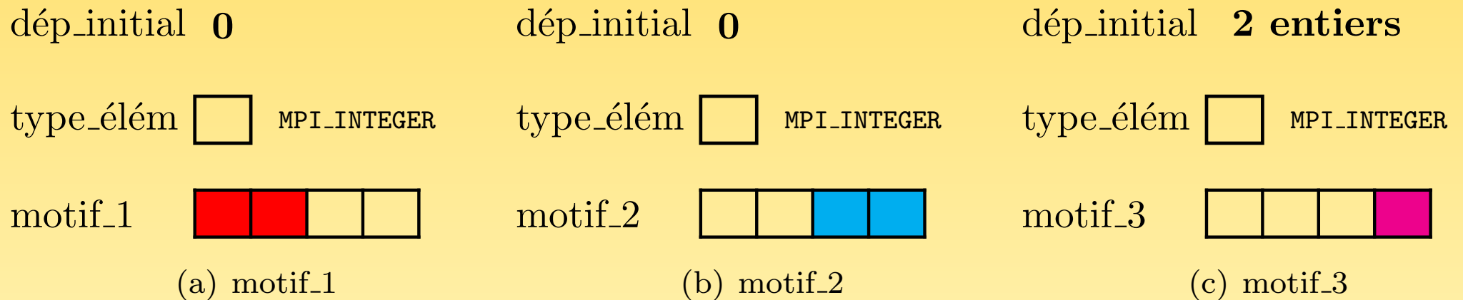
FIG. 70 – Motifs employés dans l'exemple 3 d'utilisation de MPI_FILE_SET_VIEW()
