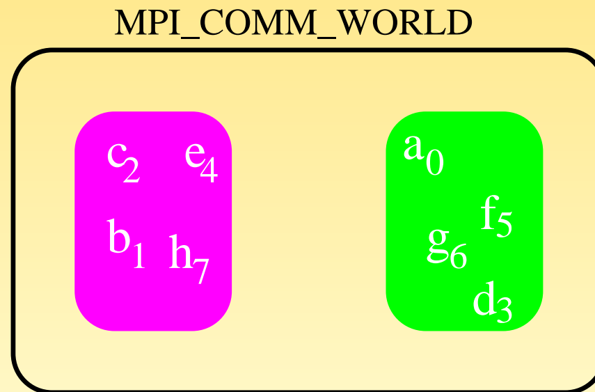
FIG. 39 – Partitionnement d'un communicateur
