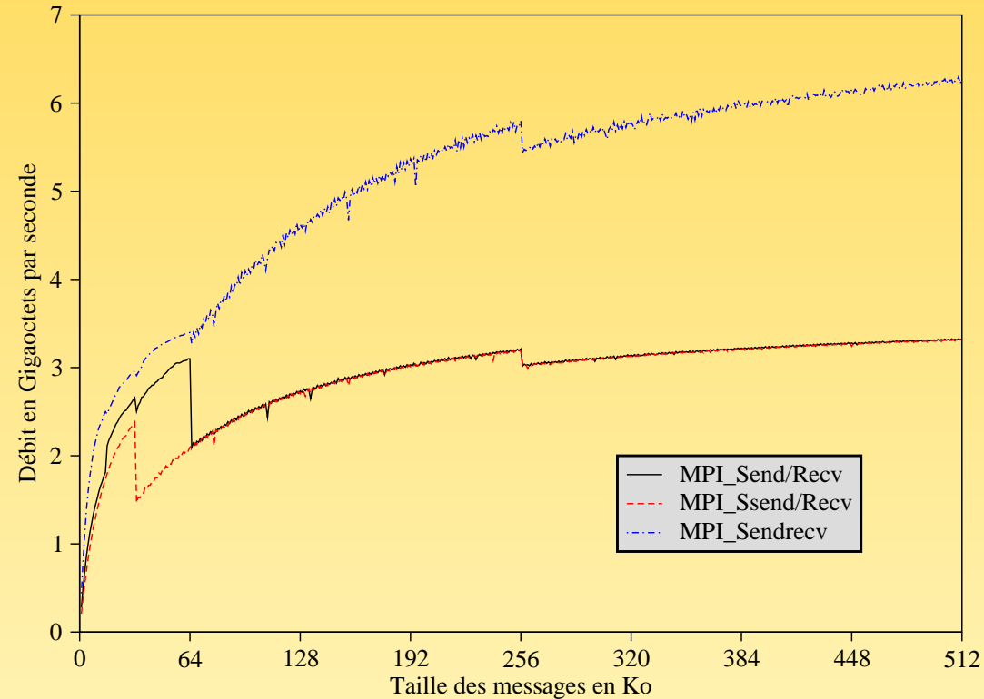
Débits des communications point à point intra-noeud sur la machine IBM P6 (MP_EAGER_LIMIT=64Ko)
