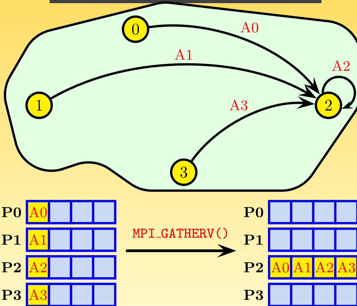
FIG. 16 – Collecte : MPI_GATHERV()
