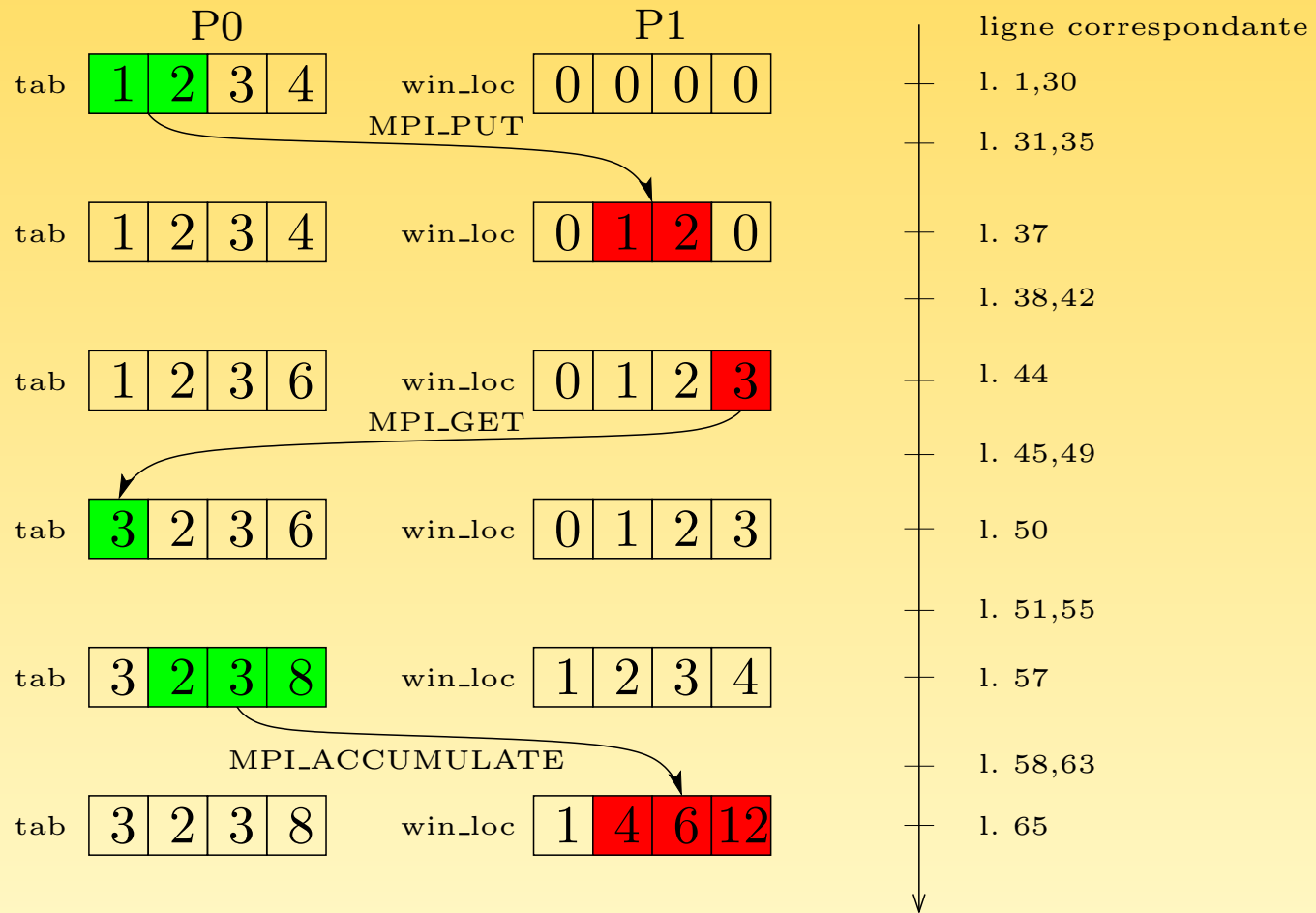
FIG. 23 – Exemple récapitulatif correspondant au code ex_fence
